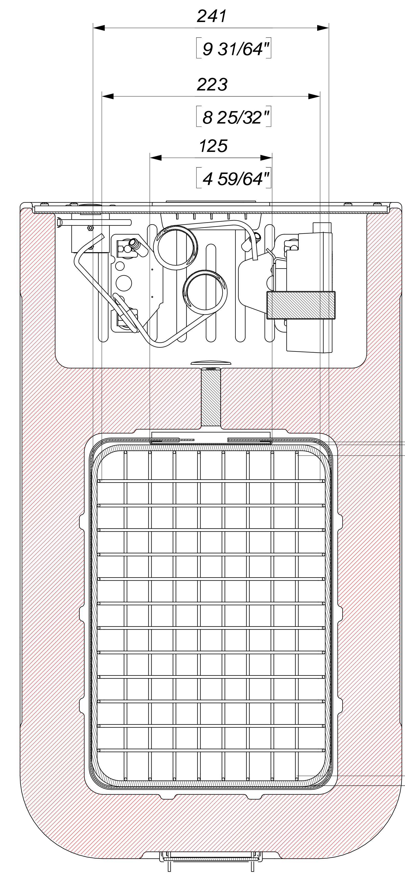
Sezione F-F SCALE 1 : 2
