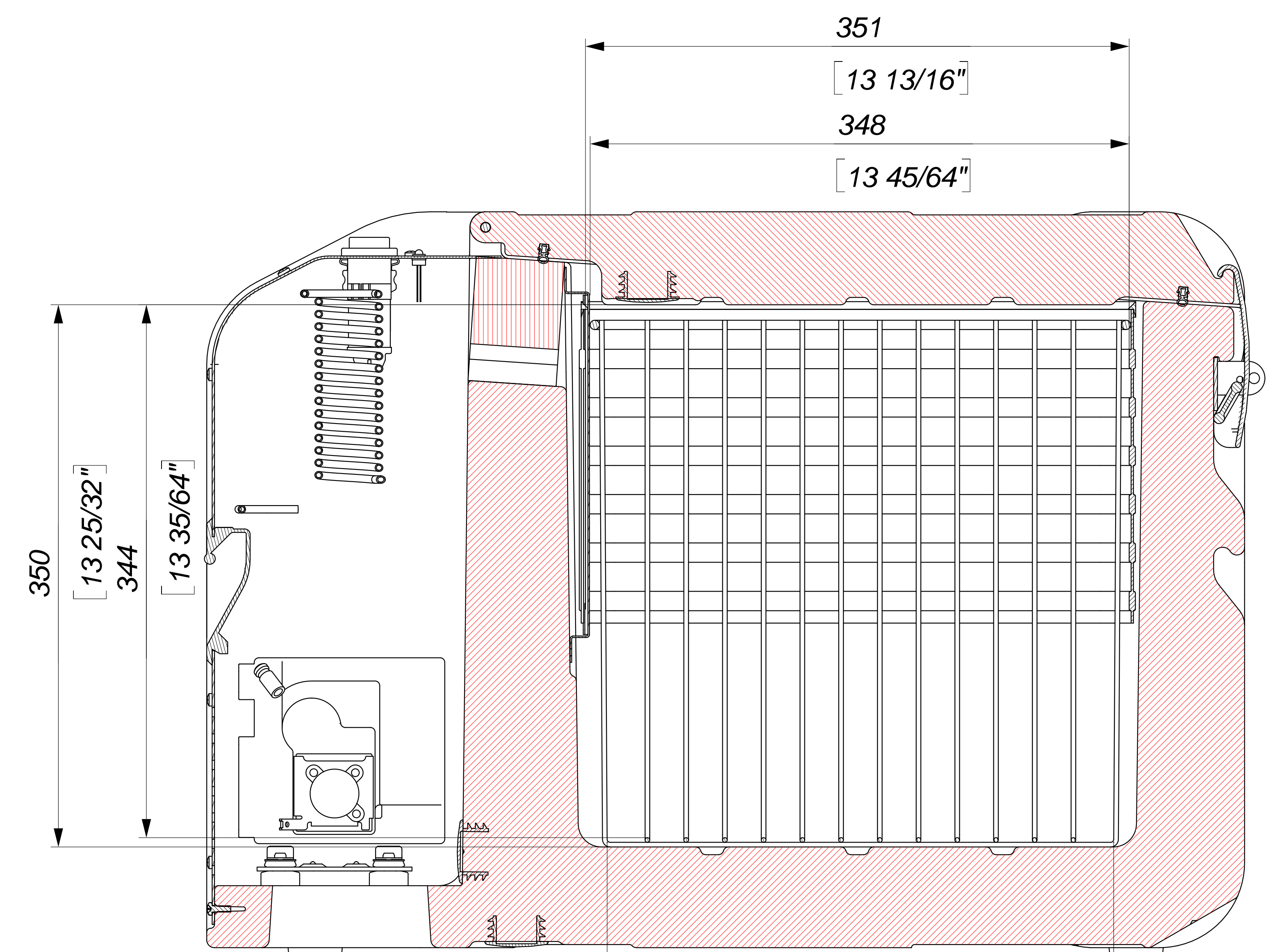
Sezione E-E SCALE 1 : 2
