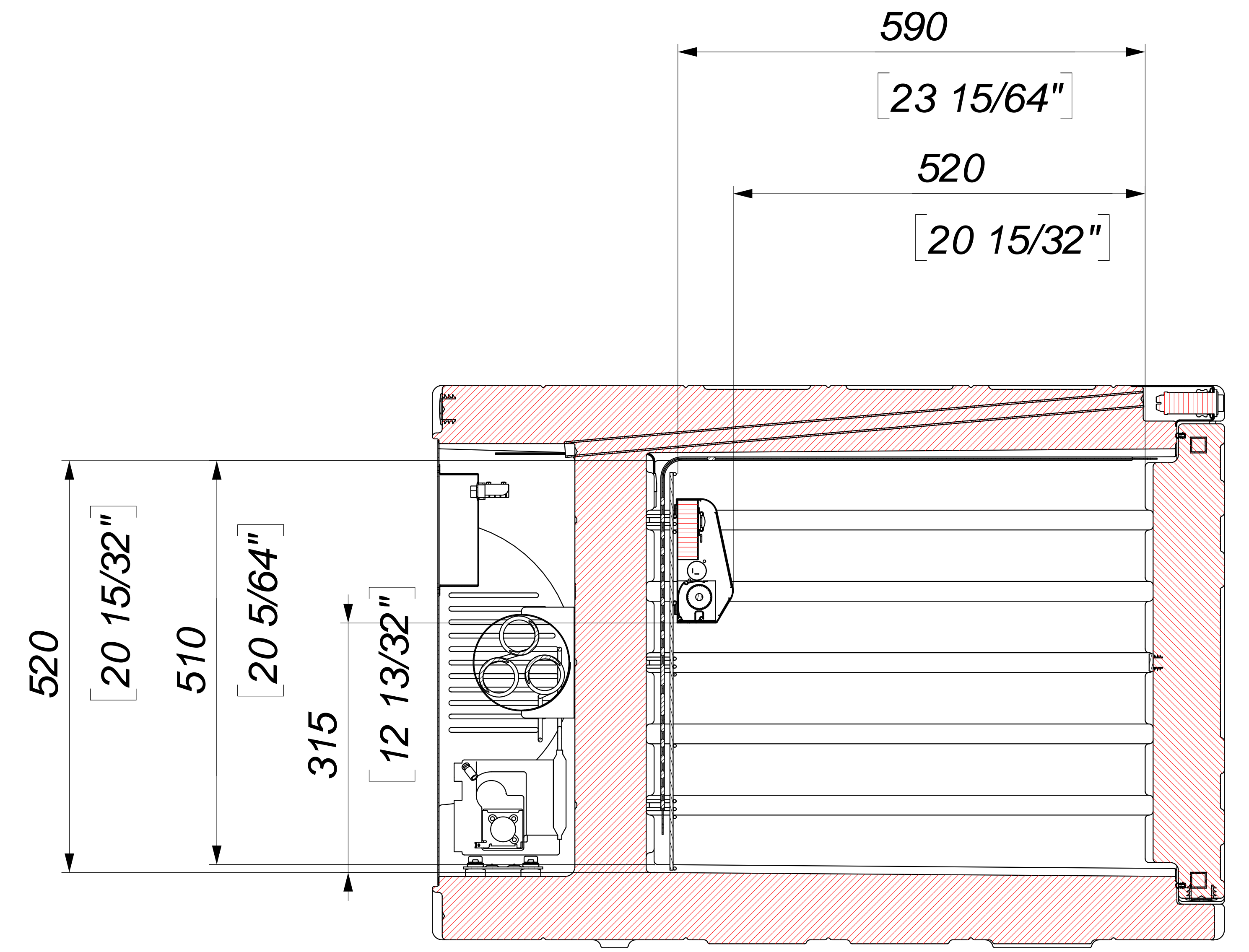
Sezione E-E SCALE 1:4
