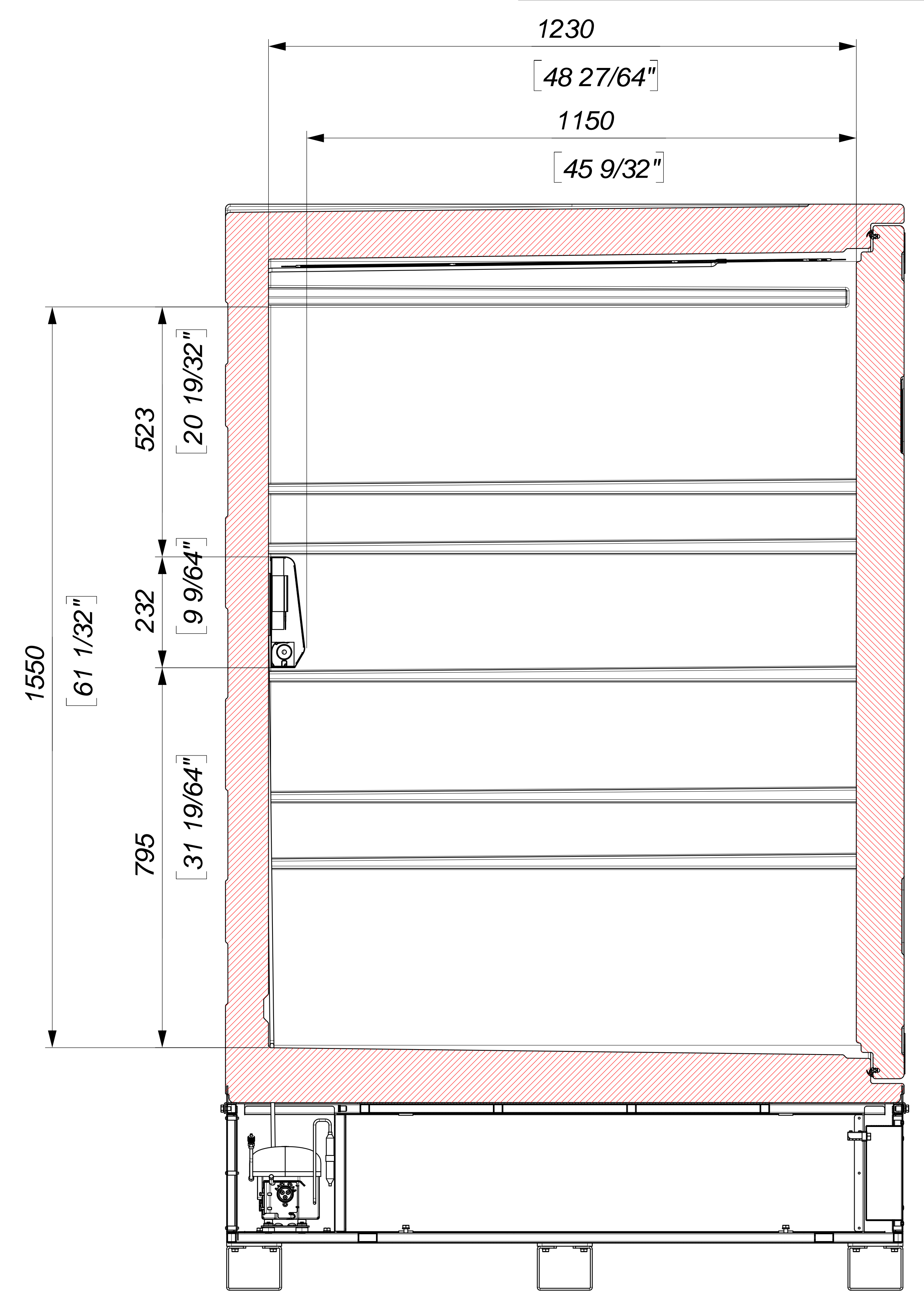
Sezione E-E SCALE 1:6
