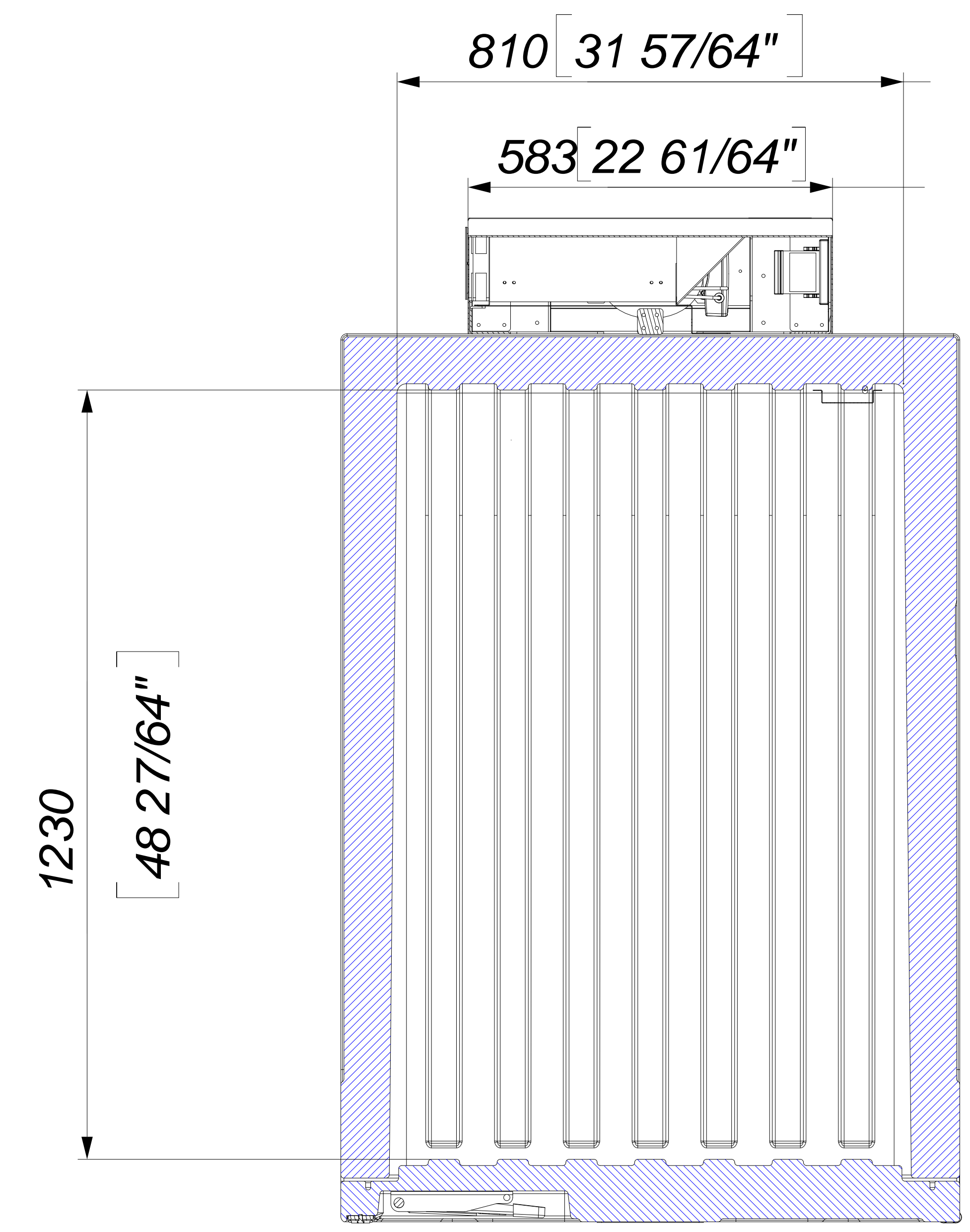
Sezione F-F SCALE 1 : 6
