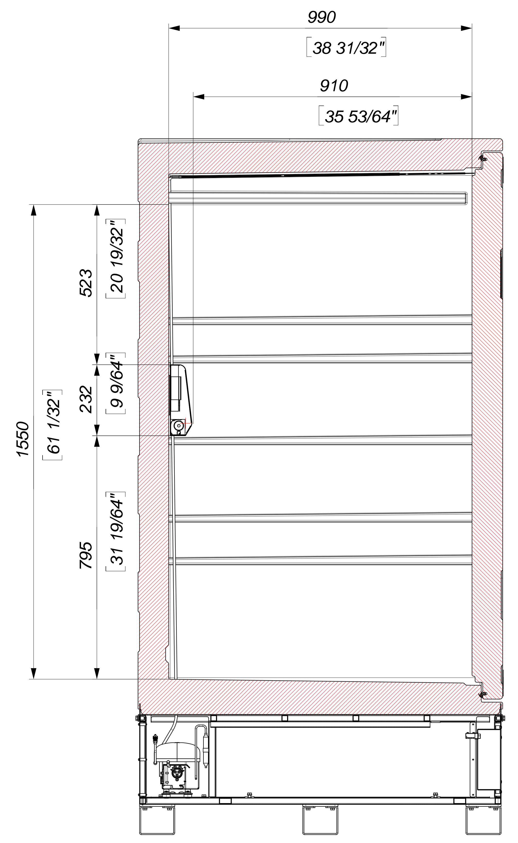
Sezione E-E SCALE 1 : 6
