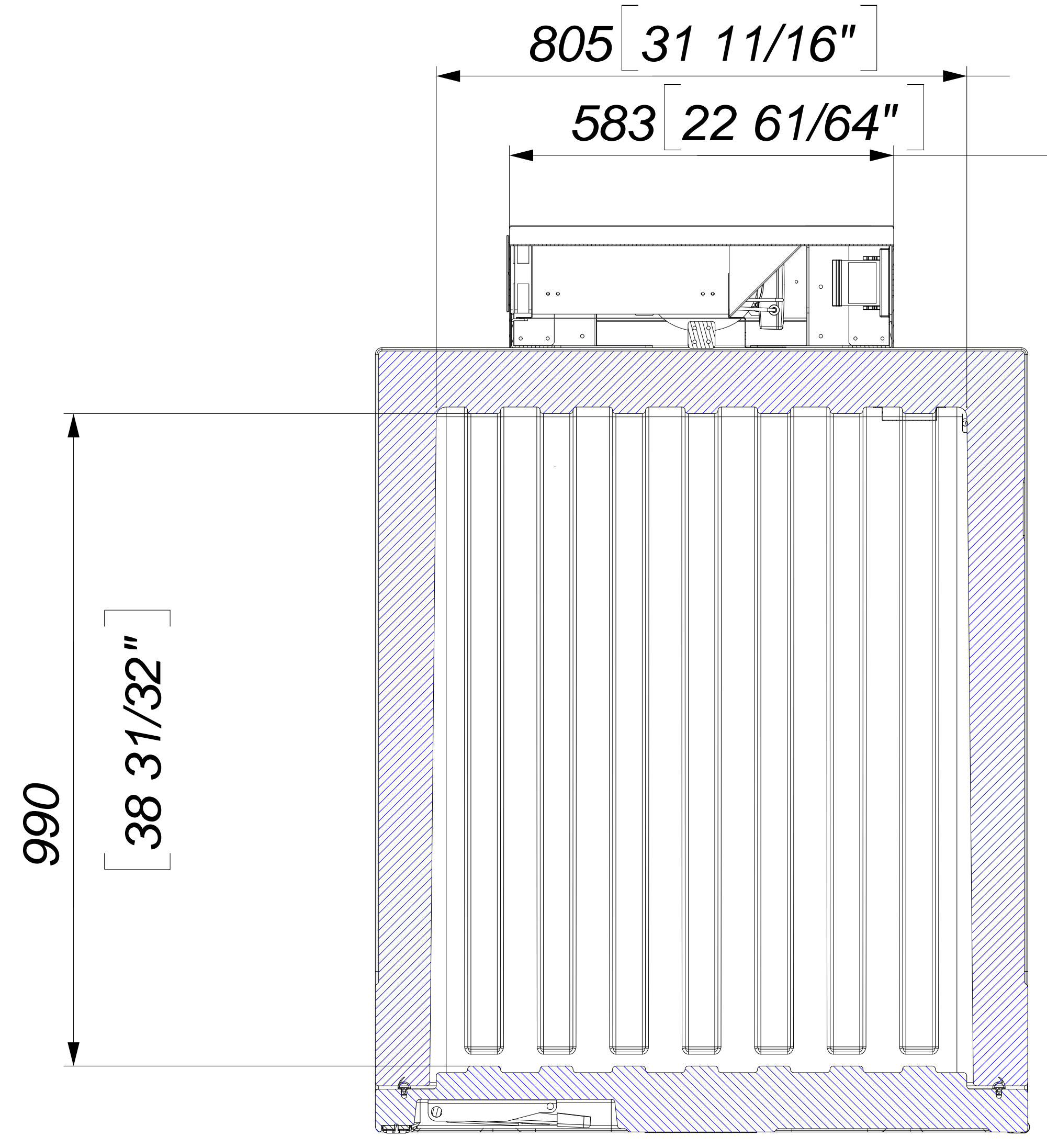
Sezione F-F SCALE 1 : 6
